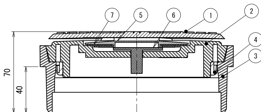
断面 A-A
