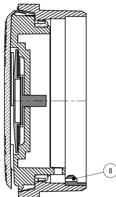
断面 B-B
